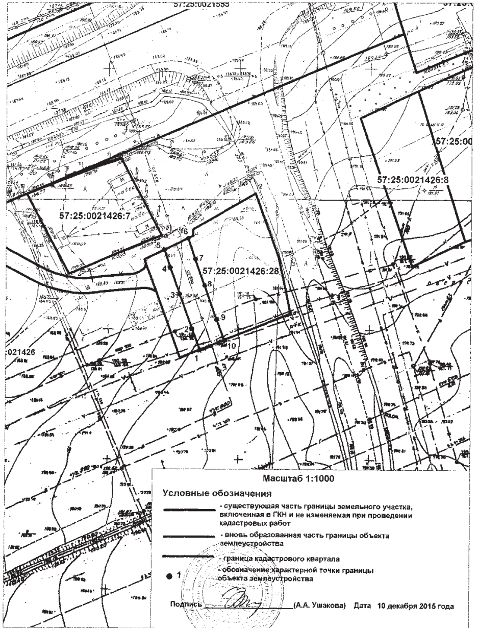
План границ объекта землеустройства "Охранная зона сети водоснабжения Ду 800 мм в границах земельного участка с кадастровым номером 57:25:0021426:28 по ул. Итальянской"
