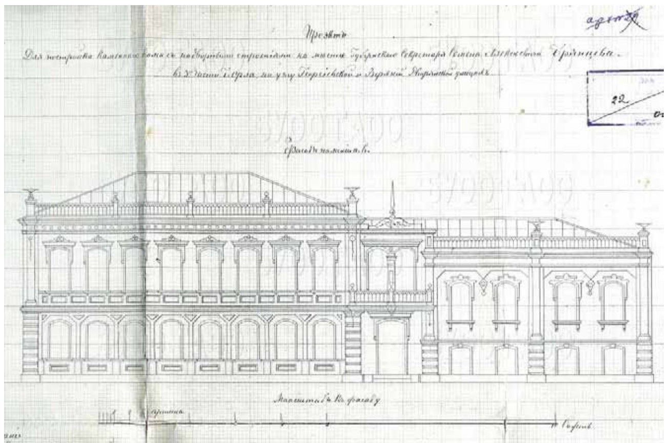
ПРОЕКТ ПОСТРОЙКИ КАМЕННОГО ДОМА С ДВОРОВЫМИ СТРОЕНИЯМИ НА МЕСТЕ ГУБЕРНСКОГО СЕКРЕТАРЯ С.А. БРЯНЦЕВА НА УГЛУ УЛИЦ ГЕОРГИЕВСКОЙ И ВЕРХНЕЙ ДВОРЯНСКОЙ В 3 ЧАСТИ Г. ОРЛА. 18 июля 1879 года. АВТОР ПРОЕКТА: ГОРОДОВОЙ АРХИТЕКТОР АКАДЕМИК И. ТИБО-БРИНИОЛЬ. ИЗ ФОНДА ГАОО.
