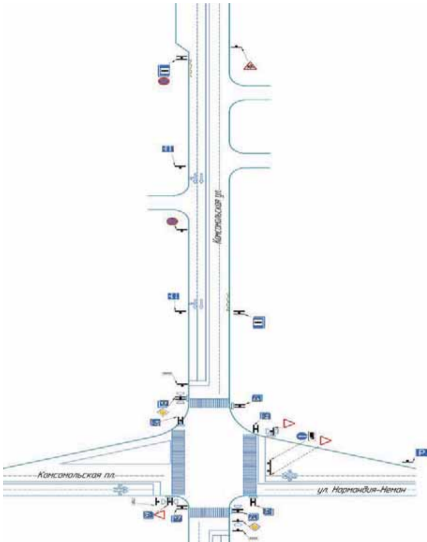
Схема установки дорожного знака 3.27 «Остановка запрещена» по ул. Комсомольской, д. № 66
