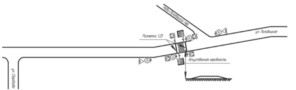
СХЕМА обустройства пешеходного перехода по ул. Половецкая города Орла
