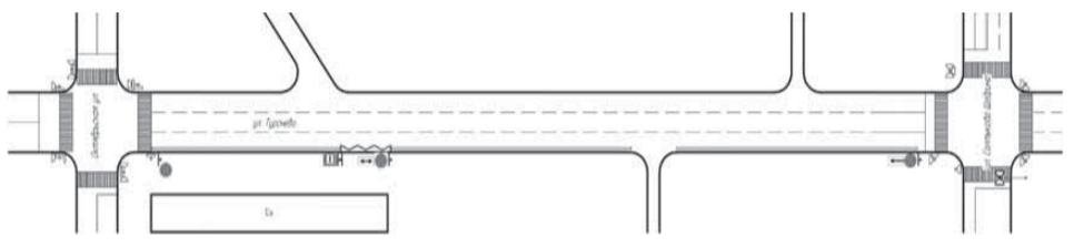
СХЕМА установки дорожных знаков 3.27 «Остановка запрещена» по четной стороне ул. Тургенева от ул. Октябрьской до ул. Салтыкова-Щедрина
