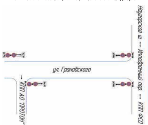
СХЕМА установки дорожных знаков 3.27 «Остановка запрещена» по ул. Грановского города Орла
