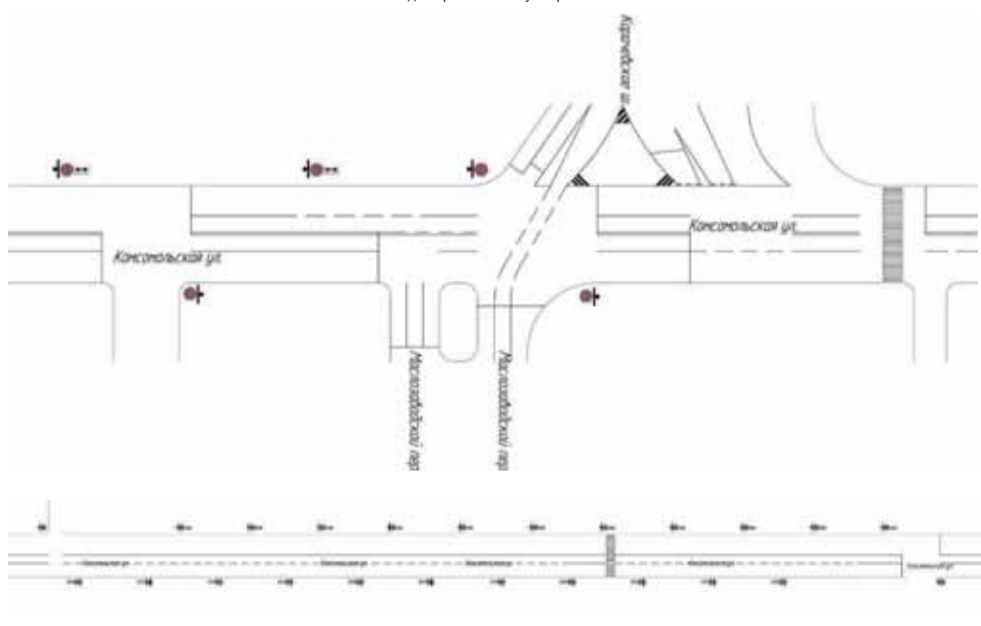
СХЕМА установки дорожных знаков 3.27 «Остановка запрещена» по ул. Комсомольская от Карачевского шоссе до пересечения с ул. Кромская
