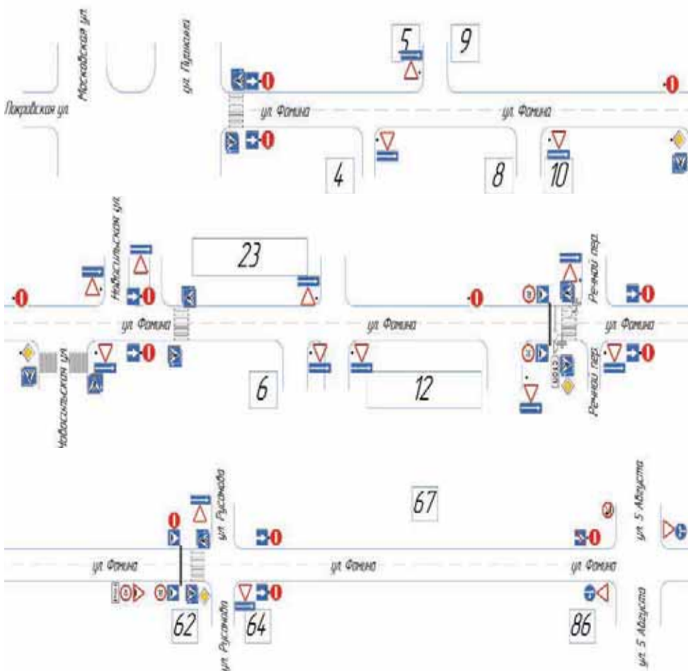
СХЕМА установки дорожных знаков по ул. Фомина от ул. Пушкина до ул. 5 Августа
