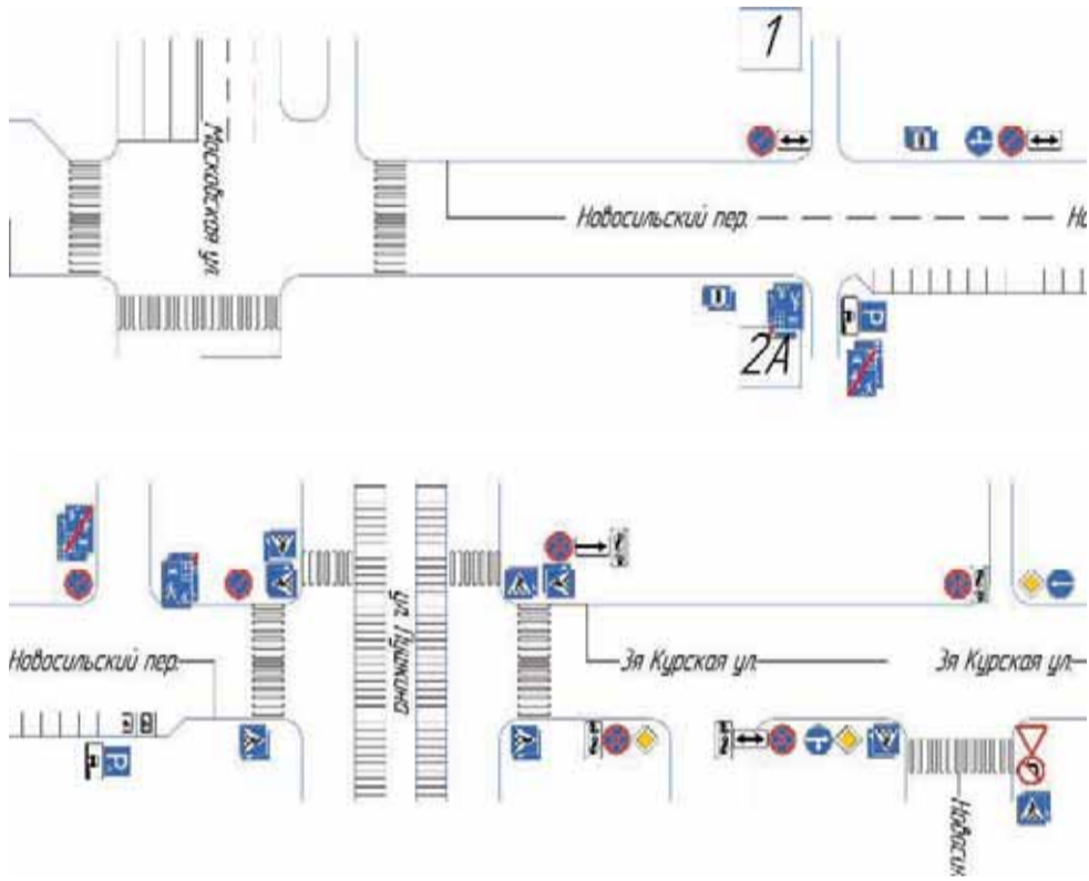
СХЕМА установки дорожных знаков по пер. Новосильский и ул. 3-я Курская
