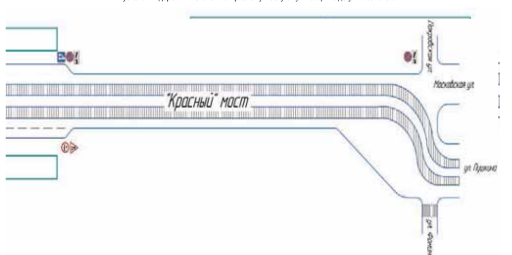
СХЕМА установки дорожных знаков по Красному мосту и ул. Гагарина до ул. Московская
