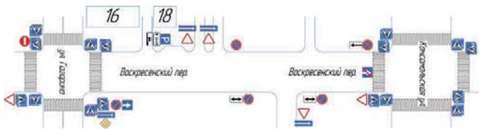
СХЕМА установки дорожных знаков по пер. Воскресенский от ул. Гагарина до ул. Комсомольская
