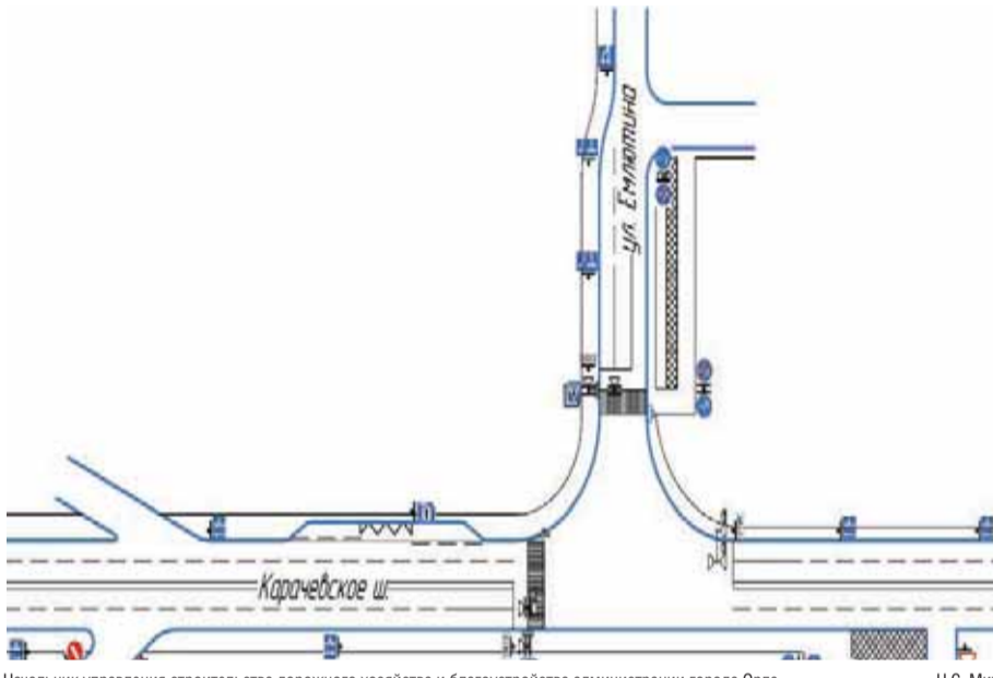
СХЕМА установки дорожных знаков по Карачевскому ш., в районе пересечения с ул. Емлютина
