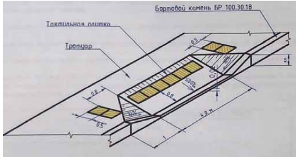
Рисунок 1 – Обустройство подхода к пешеходному переходу для мобильных групп населения
